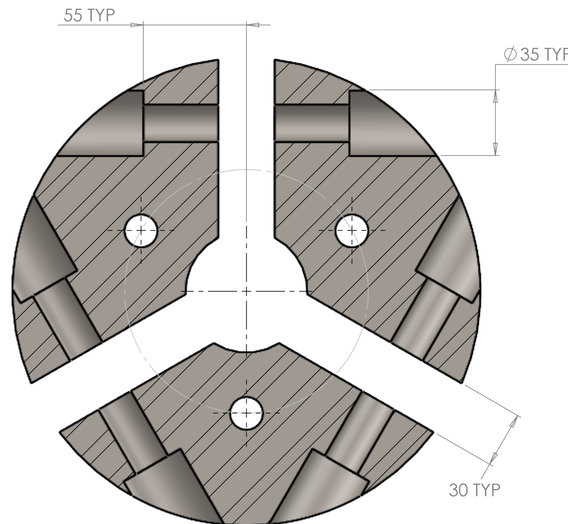
SECTION A-A
